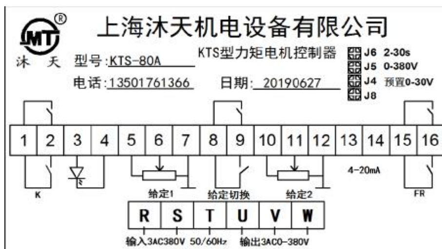
KTS 型全数字力矩电机控制器接线图
